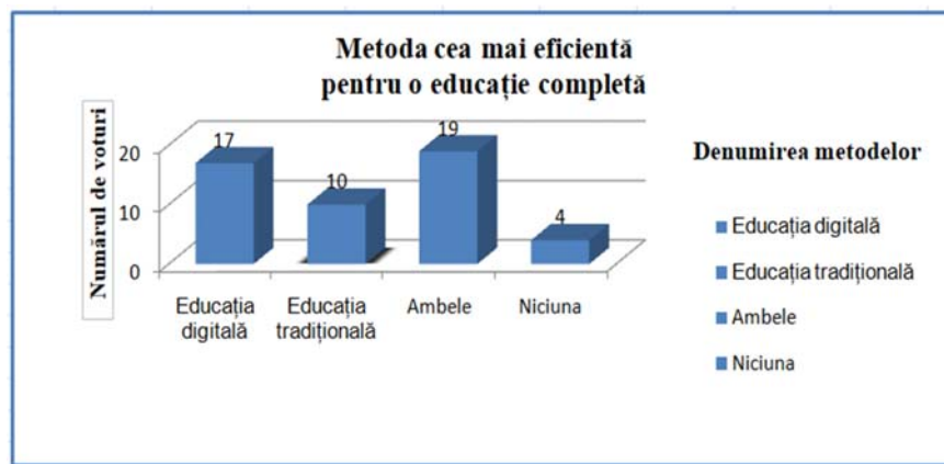
Figura 1. Rezultatele sondajului
