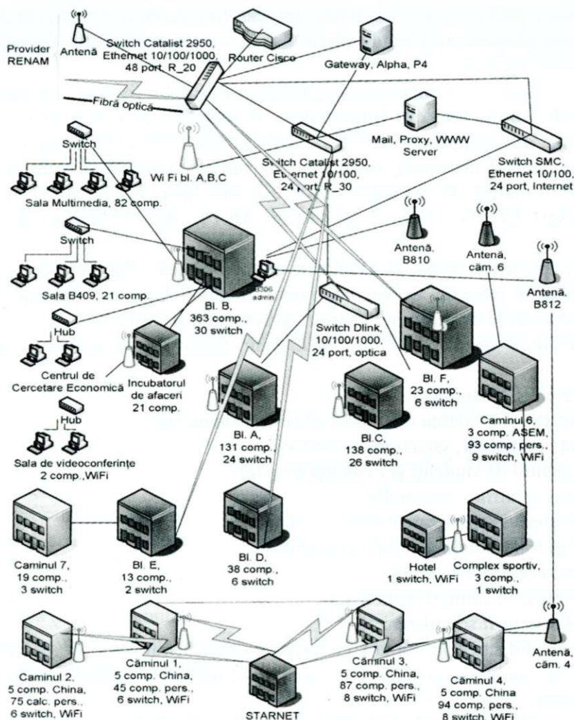
Schema Rețelei Informatice ASEM
